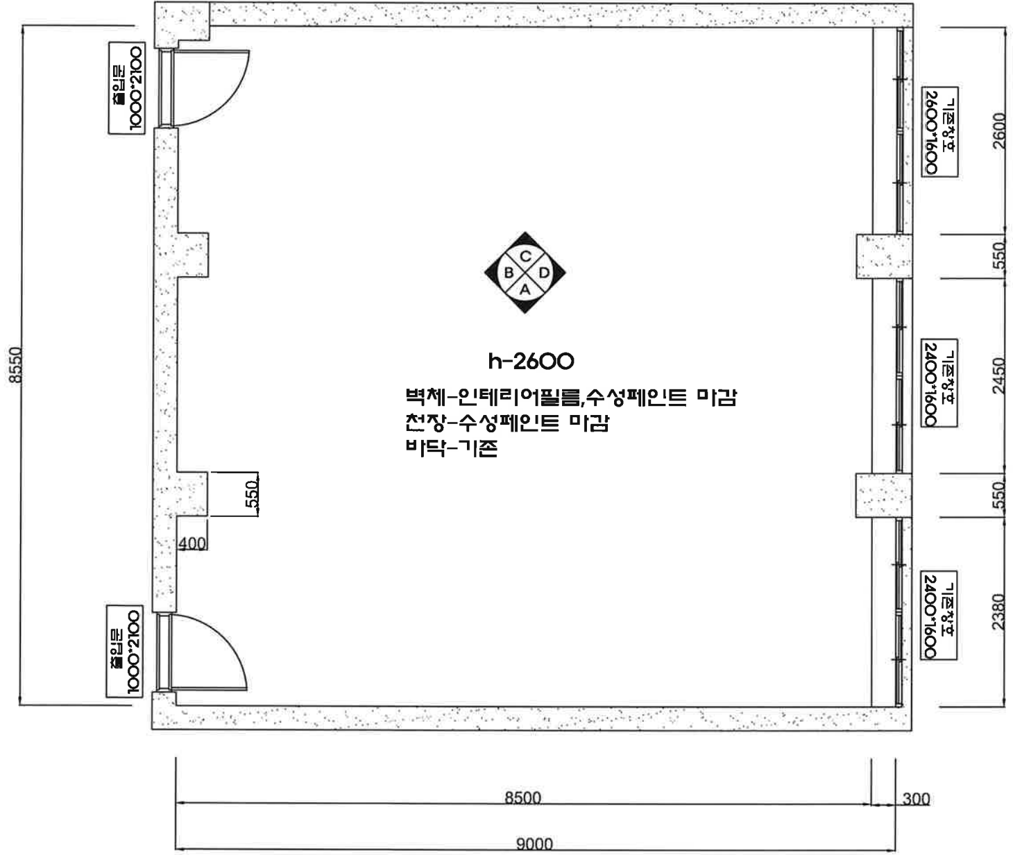
5110호 평면도 (변경 후)
