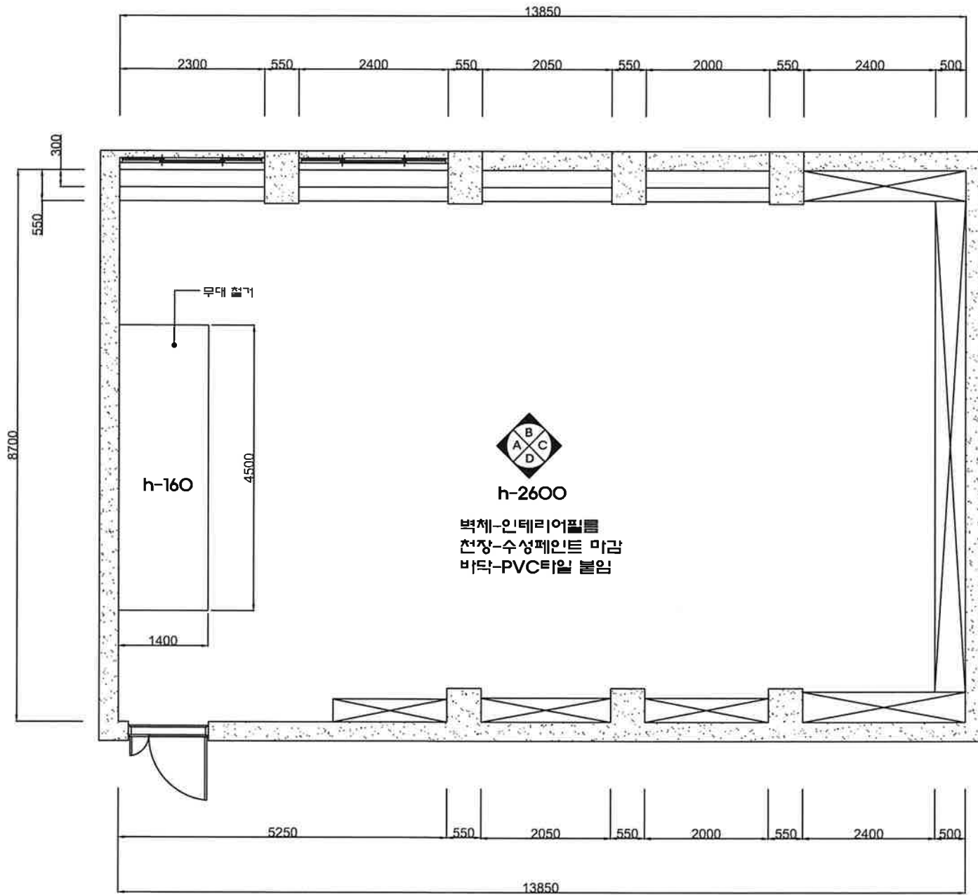
5205호 평면도 (변경 전)
