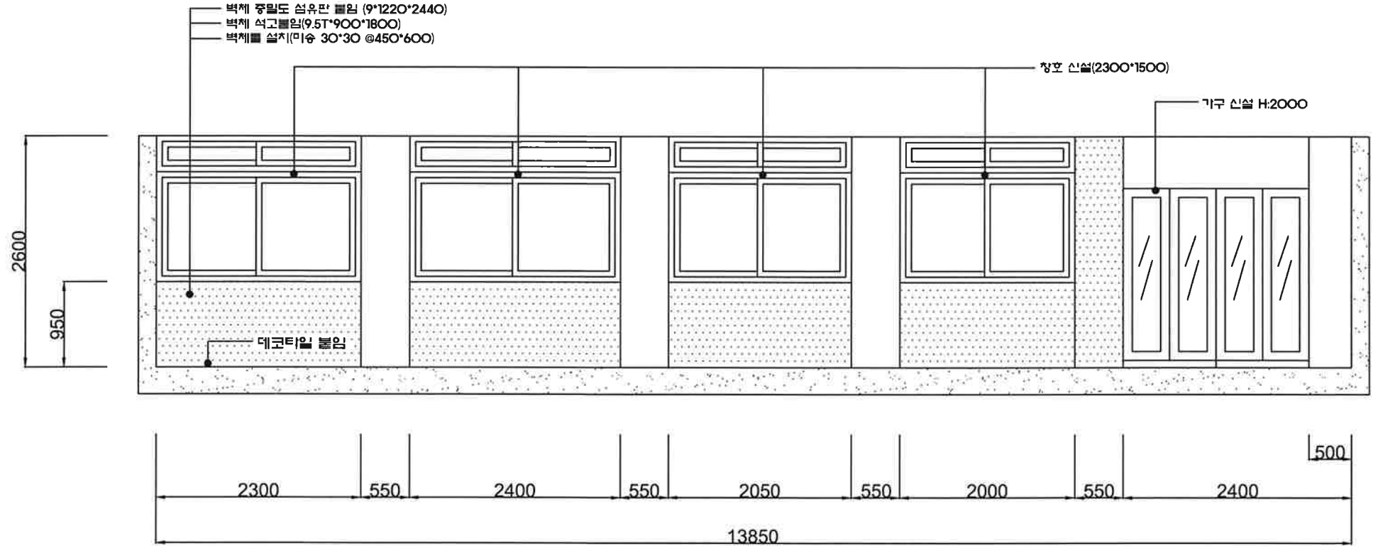
5205호 'B' 입면도(변경 후)
